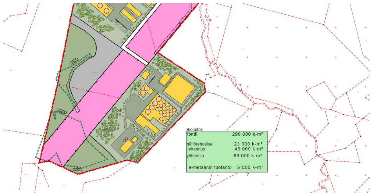
Kuva 26. Havainnollistava, esimerkin omainen kuva biokaasulaitoksen sijoittumisesta sekä tilantarpeesta alueella.
