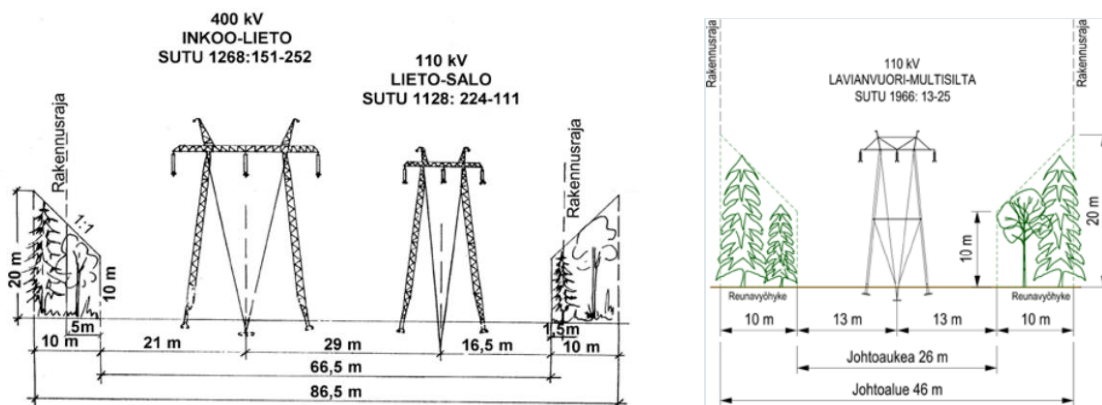
Kuva 41. Esimerkkejä voimajohtoalueen poikkileikkauksesta (Fingrid).
