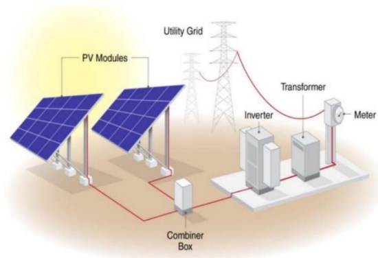
Kuva 34. Verkkoon liitetty maa-asenteinen aurinkovoimala. (kuva: NREL 2016).
